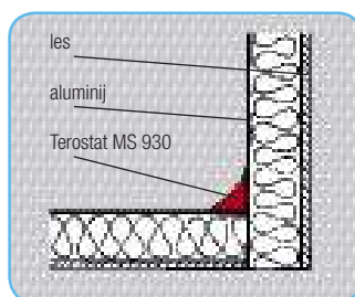
tesnjenje panelnih elementov pri hladilnih komorah
