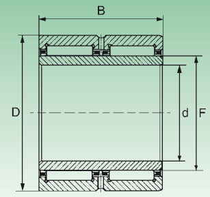
NA 69..ZW ( d \geq 32 mm)
